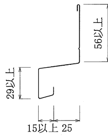
断面詳細図
