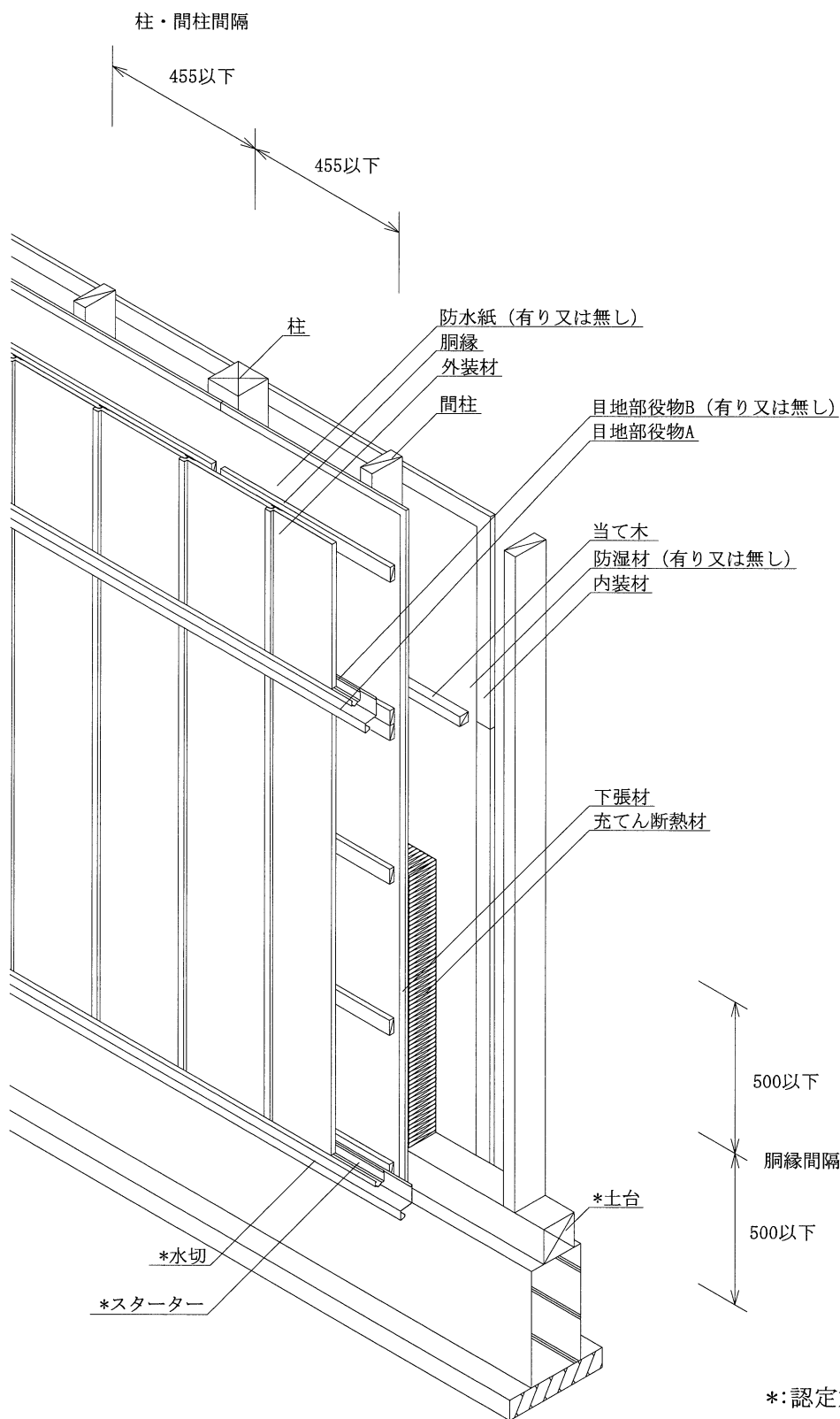
透視図 (別添 - 15)
